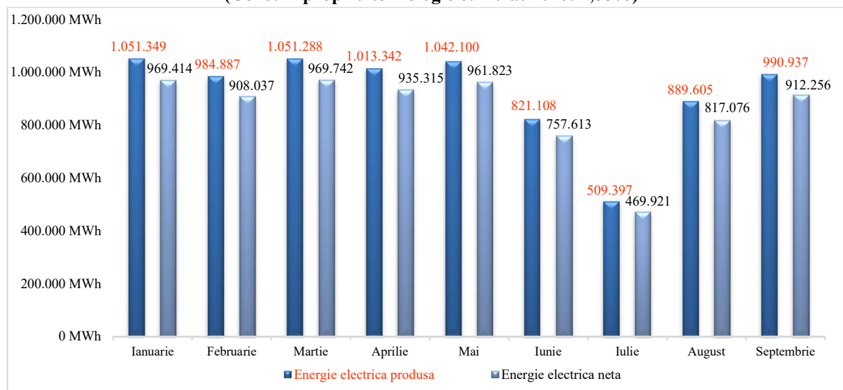
Energie electrica produsa/neta U1+U2 (MWh) (Energie electrica produsa: 8.354.013/Energie electrica neta livrata: 7.701.197) (Consum propriu tehnologic cumulat 2020: 7,88%)
